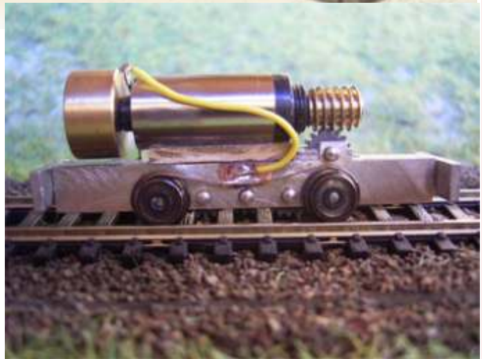
Beispielbild für das Fahrwerk Nm (hier Wismarer Schienenbus)
