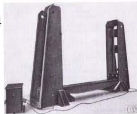
Bild 103: Spindelhebebockpaar mit Querträger
